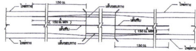
การตั้งความกว้างสะพานน้อยกว่าความกว้างจราจรตรง
