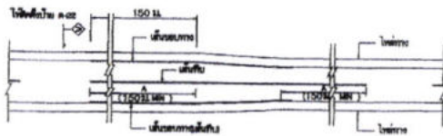
การตั้งเส้นจราจร การตั้งความกว้างของช่องจราจรตรง
