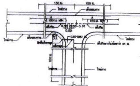
การตั้งเส้นจราจรทางตรง
