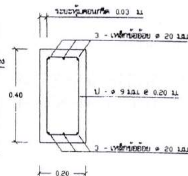
แบบขยายคาน B1 1:10
