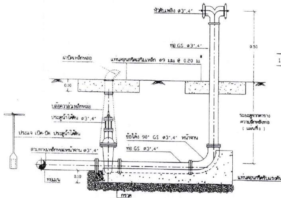
17. แบบการติดตั้งหัววัดเพลิง แบบที่ 1 1:10
