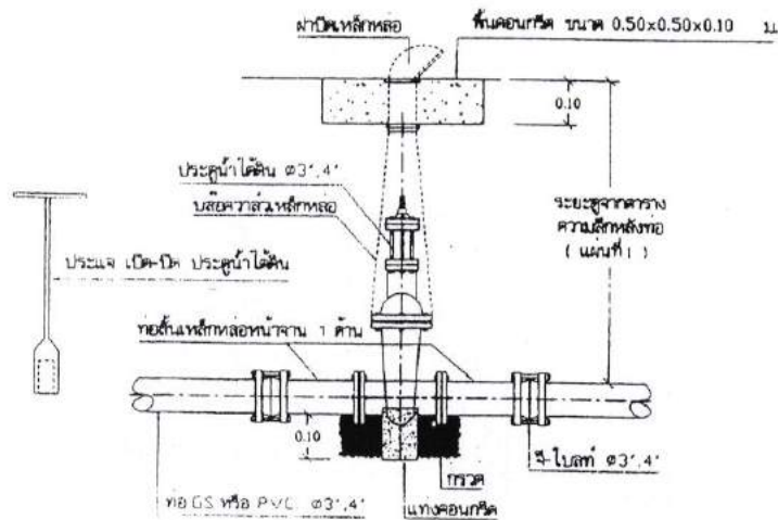
12. แผนการติดตั้งประตุน้ำใต้ดิน 1:10
