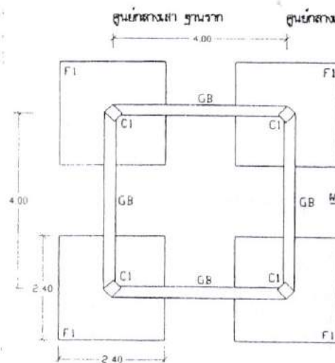
แปลนฐานราก คานคอดิน แบบไมคอกเสาเข็ม 1:75
