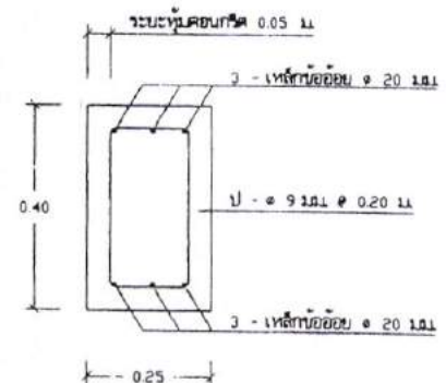
แบบขยายคาน GB 1:10
