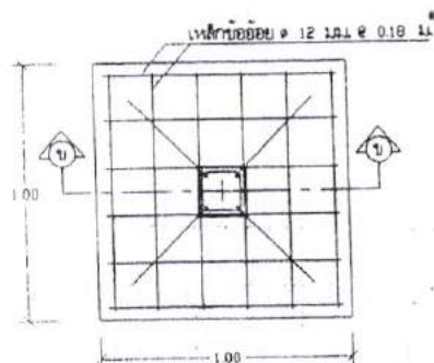
แบบขยายฐานราก F 1 : 20
