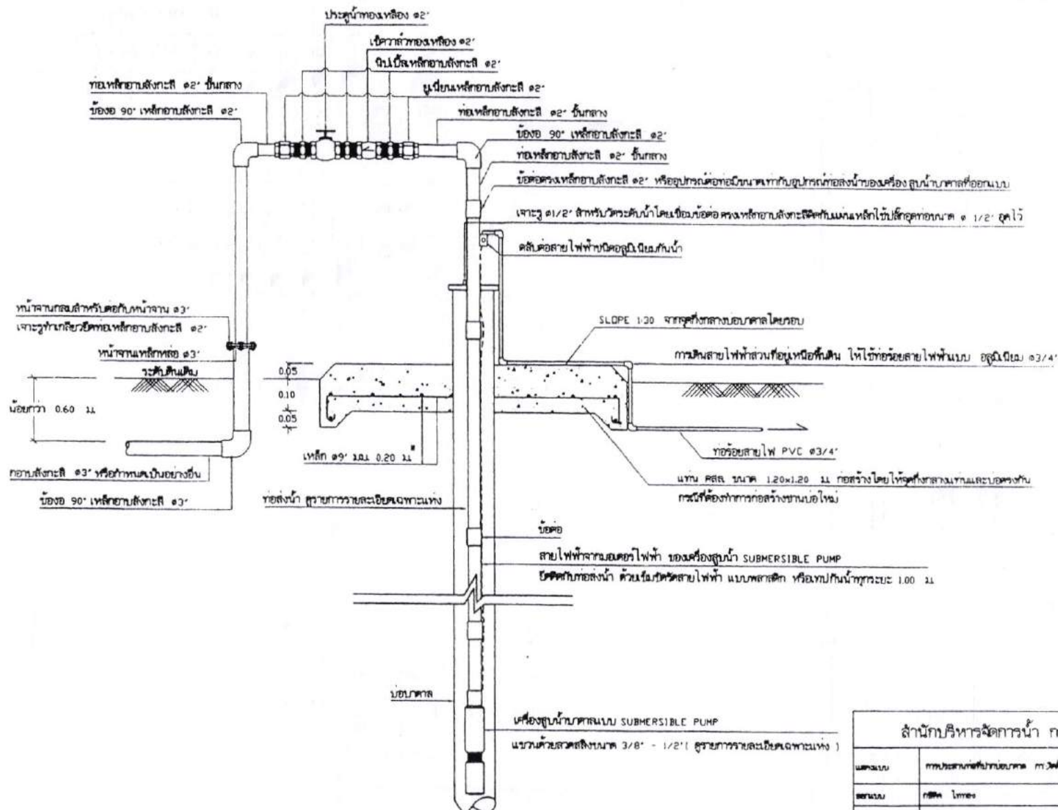
การประสานท่อที่ปากบ่อบาด การติดตั้งเครื่องสูบน้ำบาดาล แบบขับเคลื่อนไฟฟ้า 1:10
