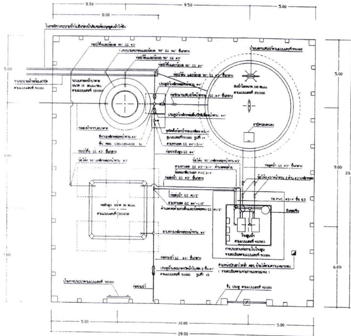
แบบการประสานท่อระหว่างระบบ (แบบมาตรฐานใหญ่) 1:100
