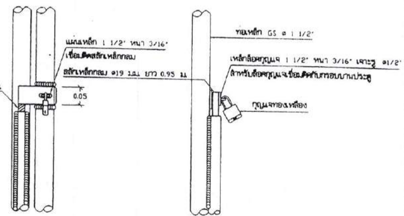
แบบขยาย สลักกลอนลือคฤญแจ 1:5
