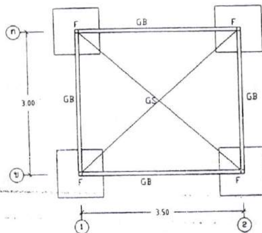
แปลนฐานราก คานคอติน แบบไม่ดัดเสาเข็ม 1 : 50
