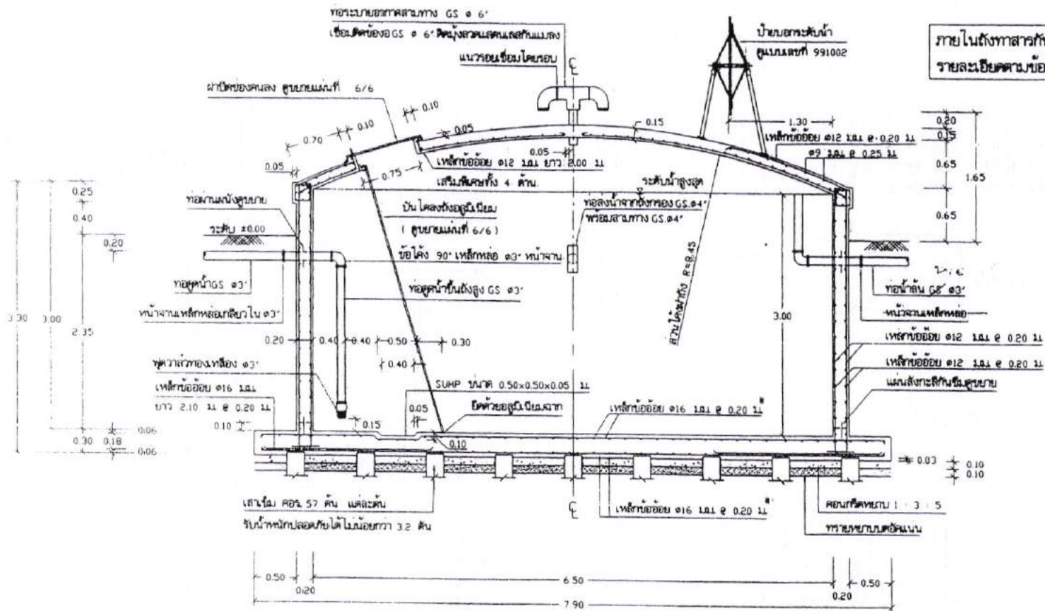
รูปตัด ก - ก 1 : 40
