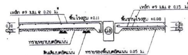
แบบขยายพื้น GS 1 : 20
