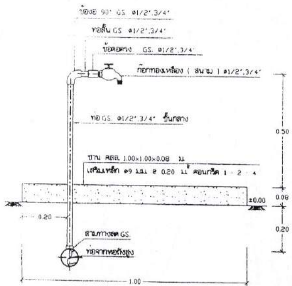
14. แผนขยายการติดตั้งก๊อกน้ำทองเหลือง 1:10
