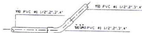
5. แบบการต่อข้อโค้ง 22 1/2".45" PVC
