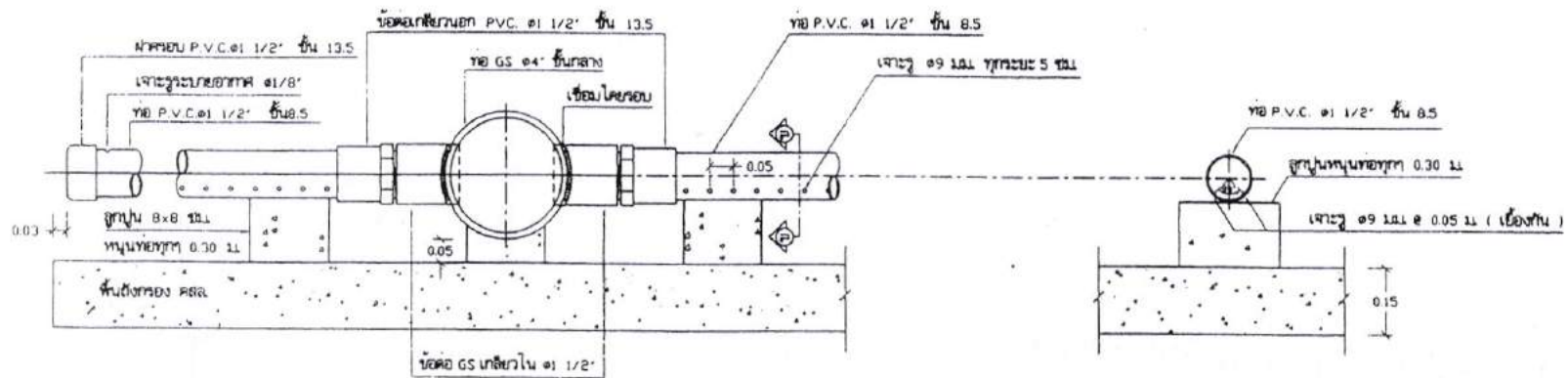
แบบขยายท่อทางปลา 1:10
