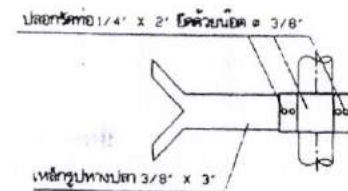
ขยายเหล็กทรงปราง 1:10
