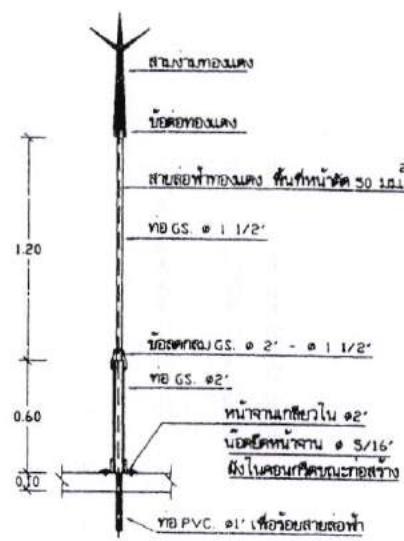
แบบขยายเสาหล่อฟ้า 1:25
